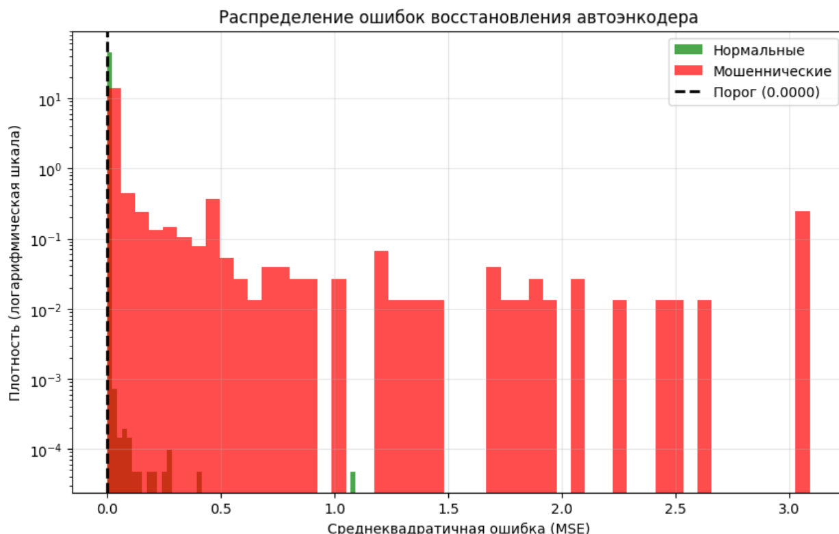
Рисунок 2. Распределение ошибок восстановления автоэнкодера
