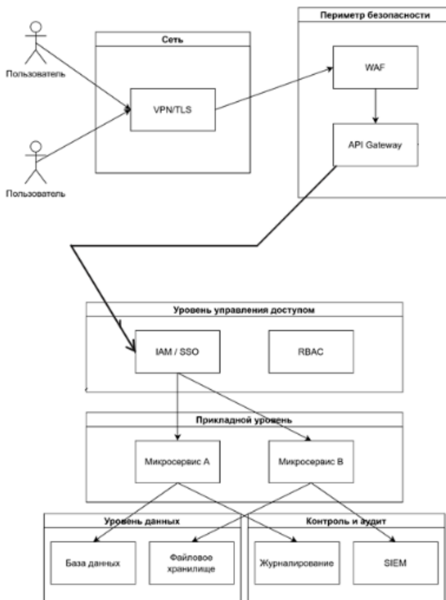
Рисунок 1. Архитектурно-логическая модель обеспечения информационной безопасности распределённой информационной системы
