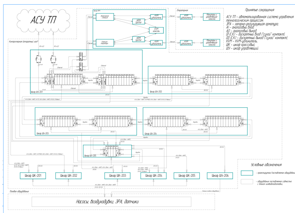
Рисунок 1 – Структурная схема ЛСУ
