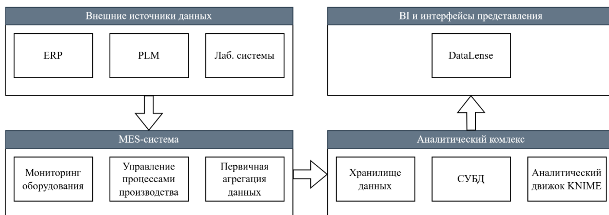
Рисунок 2. Архитектура аналитического комплекса на основе MES-системы
