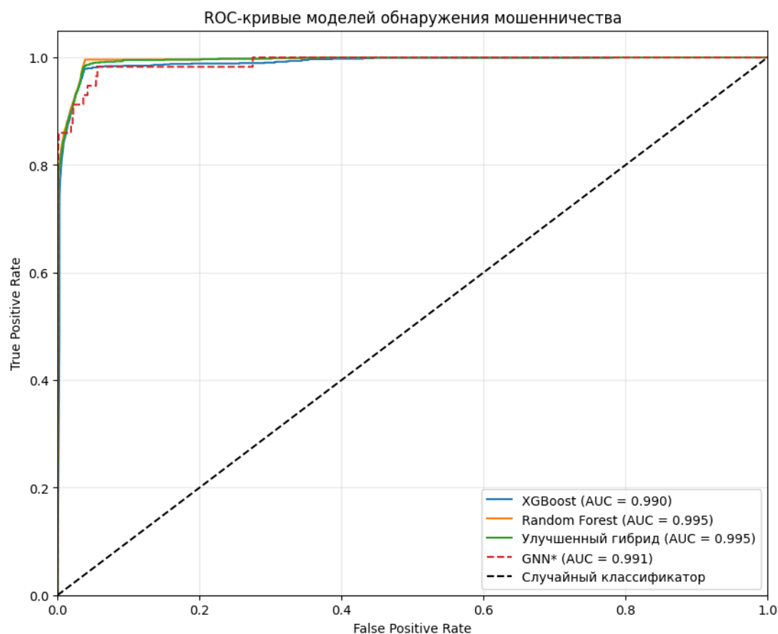
Рисунок 1. ROC-кривые моделей обнаружения мошенничества
