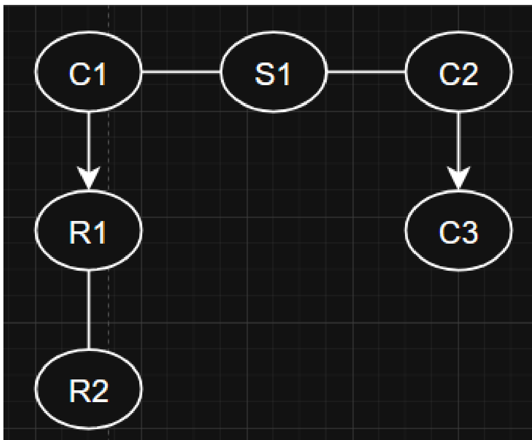
Рисунок 2 – Сетевой граф
