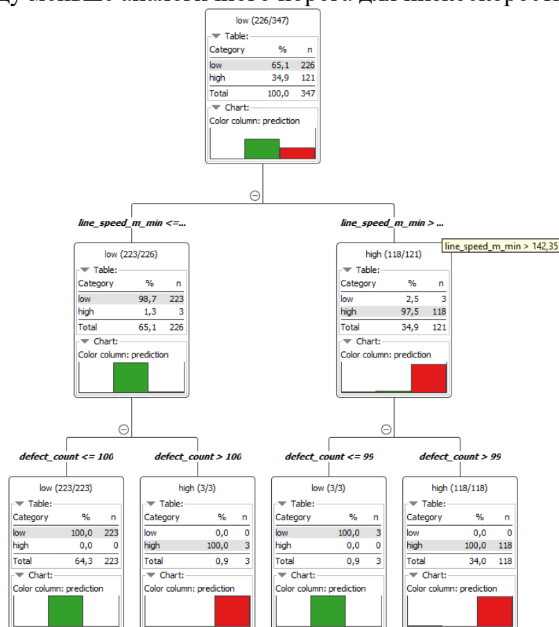
Рисунок 7. Визуализация дерева решений
