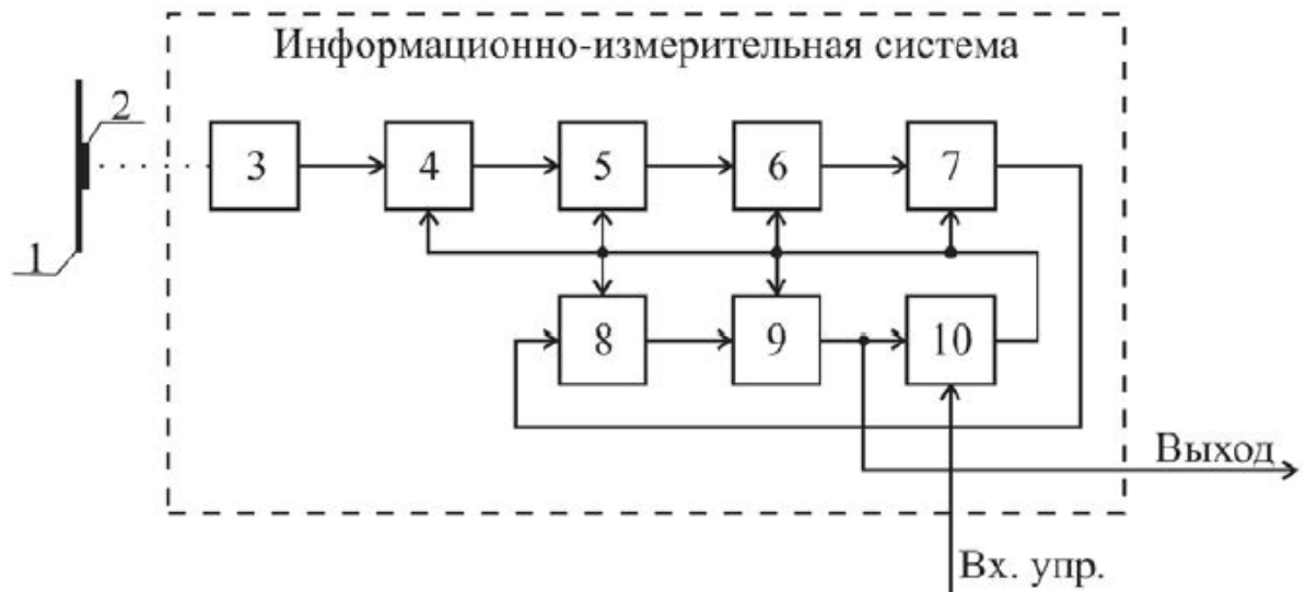
Рисунок 2 – Структура ИИС вибрационной диагностики предаварийных состояний объектов: 1 – исследуемый участок поверхности объекта контроля; 2 – тестовый объект круглой формы; 3 – регистрирующее устройство; 4 – буферный накопитель; 5 – контроллер изображений; 6 – контроллер приращений; 7 – блок статистической обработки числовых последовательностей; 8 – блок восстановления параметров вибрации; 9 – идентификатор состояний объекта контроля; 10 – устройство управления ИИС
