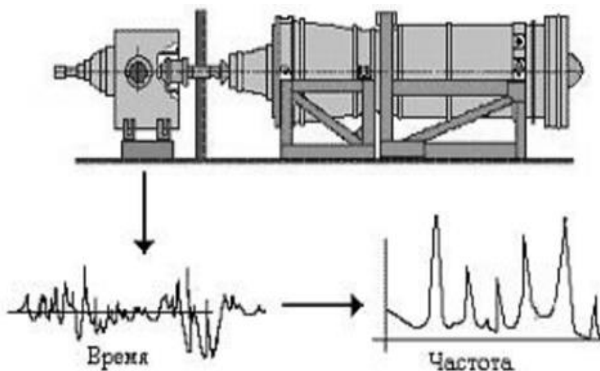
Рисунок 1 – Вибрация во временной и частотной областях
